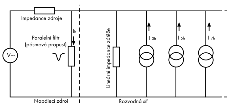
Obrázek 17 - Paralelní pasivní filtr harmonických
