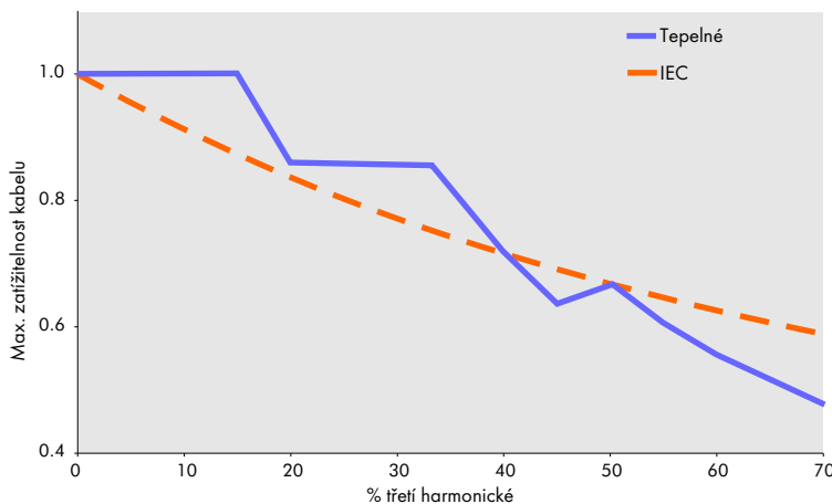
Obrázek 13 - Přepočítání zatížení kabelu pro 3n harmonickou
