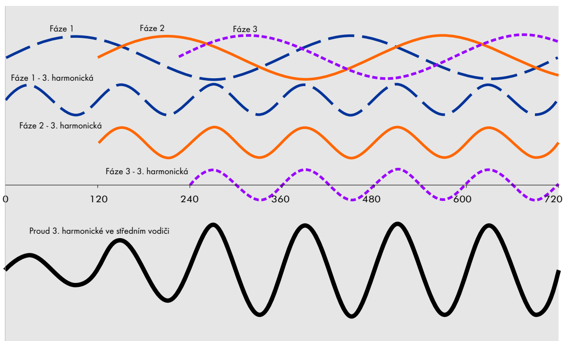
Obrázek 12 - Sčítání 3n harmonických proudů ve středním vodiči
