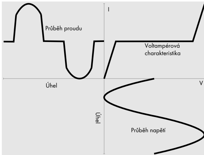
Obrázek 10 - Časový průběh proudu nelineární zátěži
