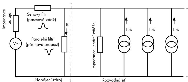
Obrázek 18 - Paralelní a sériový pasivní filtr
